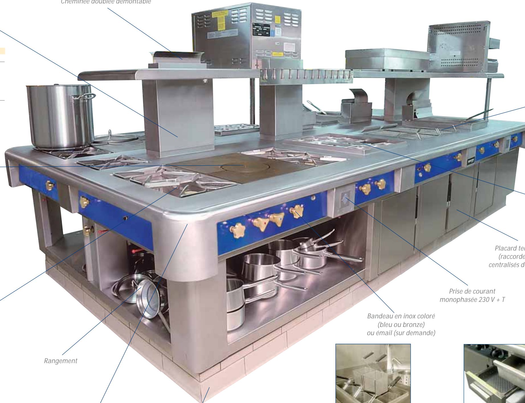
Cheminée doublée démontable
