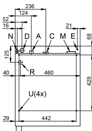
Position de raccordement fond de l'appareil
