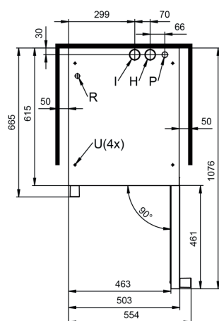
Vue de dessus avec distances aux murs
